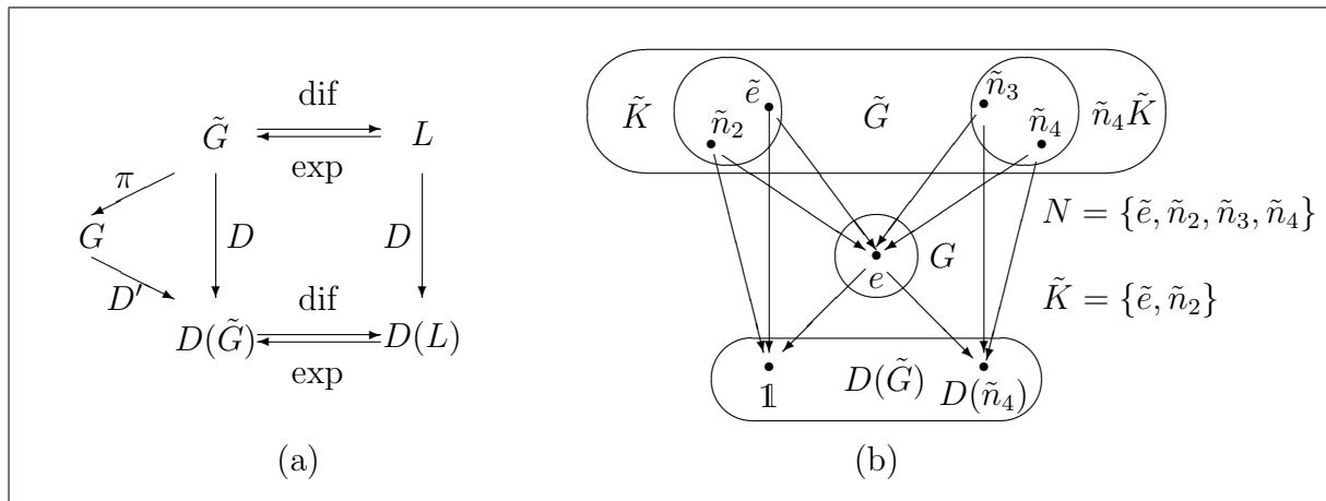
Slika 5.2: Veza reprezentacija grupa i algebri. (a) Svaka reprezentacija D' grupe G je i reprezentacija D = D' \circ \pi grupe \tilde{G} , i diferenciranjem daje reprezentaciju algebre; u suprotnom smeru, eksponenciranjem se dobija samo reprezentacija \tilde{G} . (b) Višeznačne reprezentacije.
