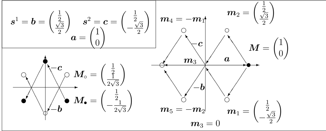
Slika 4.5: \mathfrak{sl}(3, \mathbb{C}) : fundamentalne ( M_o = \begin{pmatrix} \frac{1}{2} \\ \frac{1}{2\sqrt{3}} \end{pmatrix} i M_\bullet = \begin{pmatrix} \frac{1}{2} \\ -\frac{1}{2\sqrt{3}} \end{pmatrix} ) i pridružena reprezentacija.
