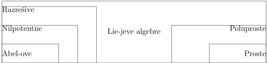
Slika 4.1: Podela Lie-jevih algebri.
