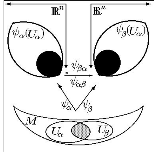
Slika 1.2: Karte na mnogostrukosti.
