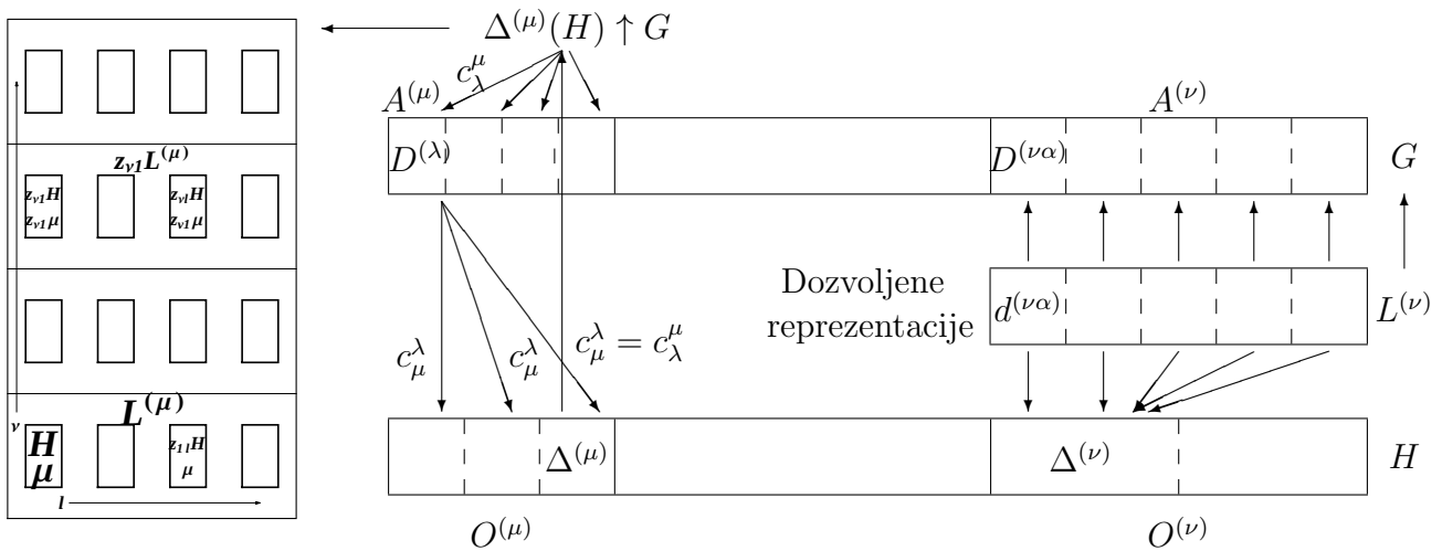
Slika 3.6: Indukcija sa invarijantne podgrupe. Levo: Koseti podgrupe H grupisani u podgrupu L^{(\mu)} (donji red, koji G -konjugacijom daju reprezentacije ekvivalentne sa \Delta^{(\mu)}(H) ) i njene kosete (neekvivalentne reprezentacije). Sredina i desno: Donji i gornji pravougaonik su skupovi neekvivalentnih ireducibilnih reprezentacija grupa H , odnosno G , podeljeni na orbite G -konjugacije, odnosno asocirane skupove. Srednji deo slike ilustruje teorem 3.21: ireducibilne komponente indukovane reprezentacije su iz jednog asociranog skupa. Desno je prikazana konstrukcija asociranog skupa preko dozvoljenih reprezentacija male grupe (teorem 3.22).
