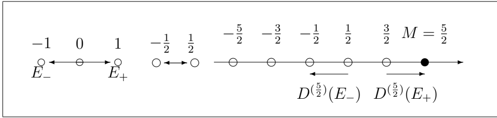
Slika 4.4: \mathfrak{sl}(2, \mathbb{C}) : korenovi i težine pridružene (ireducibilna sa M = 1 ), fundamentalne ( M = \frac{1}{2} ) i reprezentacije M = \frac{5}{2} .
