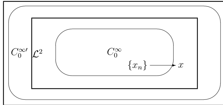
Slika 2.1: Konstrukcija Lebesgue-ovog prostora. Cauchy-jev niz \{x_n\} iz C_0^\infty konvergira ka x iz C_0^{\infty'} , pa je x iz \mathcal{L}^2 .
