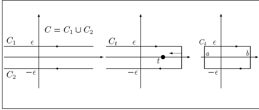
Slika 2.4: Kontura integracije za autoadjungovani operator. Levo: spektralna forma (2.7); sredina: neprekidnost projektorske mere (2.8); desno: projektor intervala. Svuda je \epsilon > 0 .
