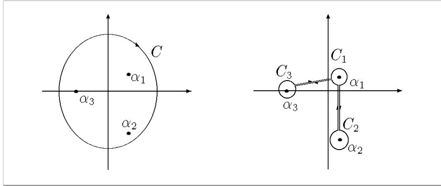
Slika 2.3: Sažimanje konture integracije oko svojstvenih vrednosti.
