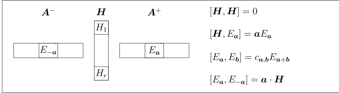
Slika 4.2: Standardna forma poluproste algebre.
