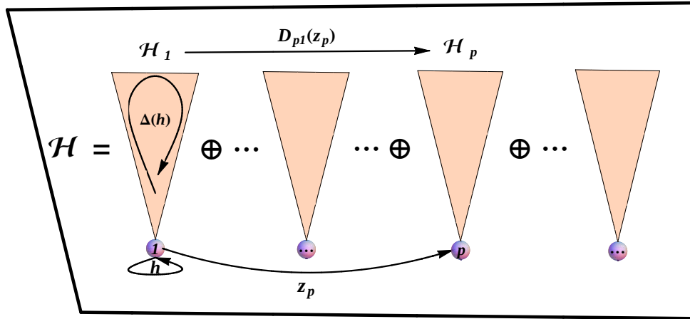
Slika 3.5: Geometrija indukcije. Osnovno dejstvo (osnova slike) na nekoj orbiti sa stabilizatorom H (elementi h ), odnosno grupno množenje kad se tačke orbite identifikuje sa transversalom (elementi z_p ), "podigne" se u vektorski prostor \mathcal{H} koji je raslojava u direktni zbir potprostora (slojeva) nad tačkama orbite.
