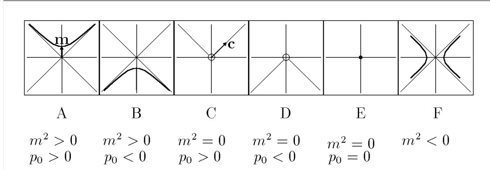
Slika 5.3: Orbite reprezentacija grupe T^4 pri dejstvu Poincaré-ove grupe. Dat je presek u ravni p_0 p_3 , pri čemu je osa p_0 usmerena naviše, a p_3 nadesno. Cele orbite se dobijaju delovanjem prostornih rotacija na ove preseke, tj. ortogonalnim transformacijama koje ostavljaju p_0 -osu invarijantnom. Kod fizički značajnih orbita A i C, pokazani su predstavnici orbita \mathbf{m} = (m, 0, 0, 0)^T i \mathbf{c} = (1, 0, 0, 1)^T .
