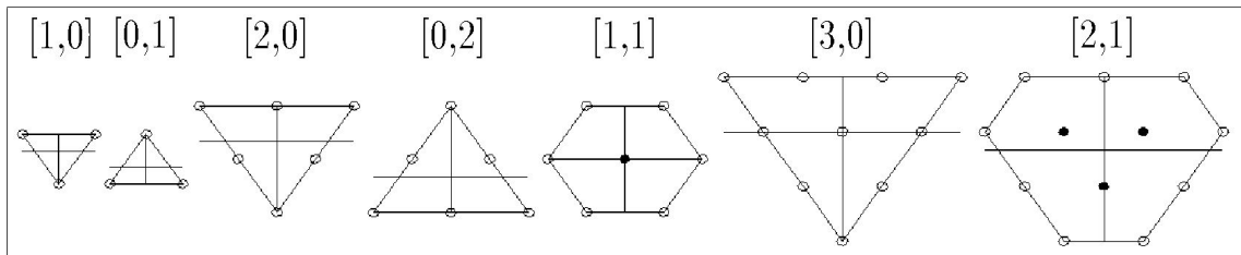
Slika D.2: Dijagrami težina za reprezentacije \mathfrak{sl}(3, \mathbb{C}) .
