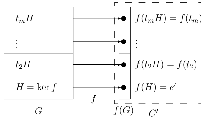
Slika 3.2: Struktura homomorfizma. Lik f(G) homomorfizma f izomorfan je faktor grupi G/\ker f .
