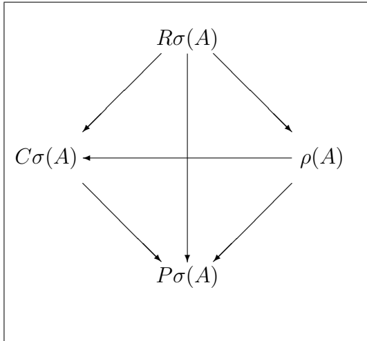
Slika 2.2: Promena delova spektra pri proširenju operatora.
