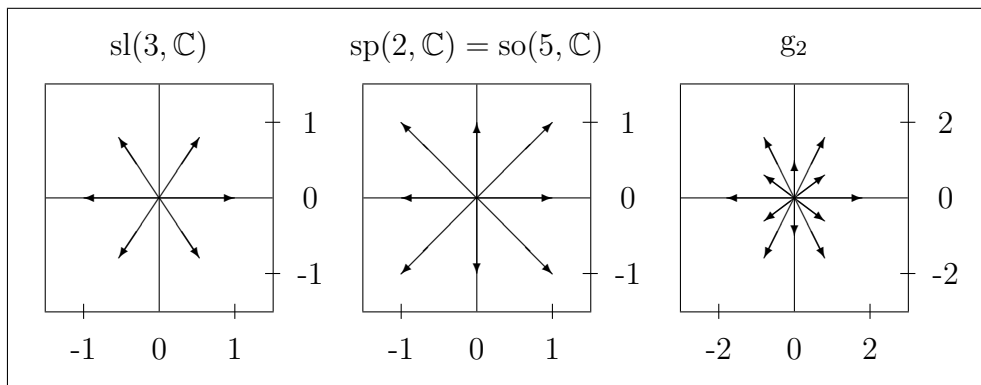
Slika D.3: Koreni sistemi prostih algebri ranga 2.
