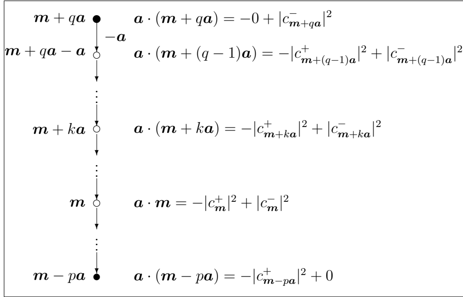
Slika 4.3: \mathbf{a} -niz iz \mathbf{m} .
