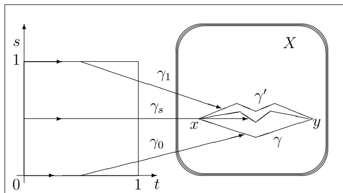
Slika 1.1: Homotopni putevi.
