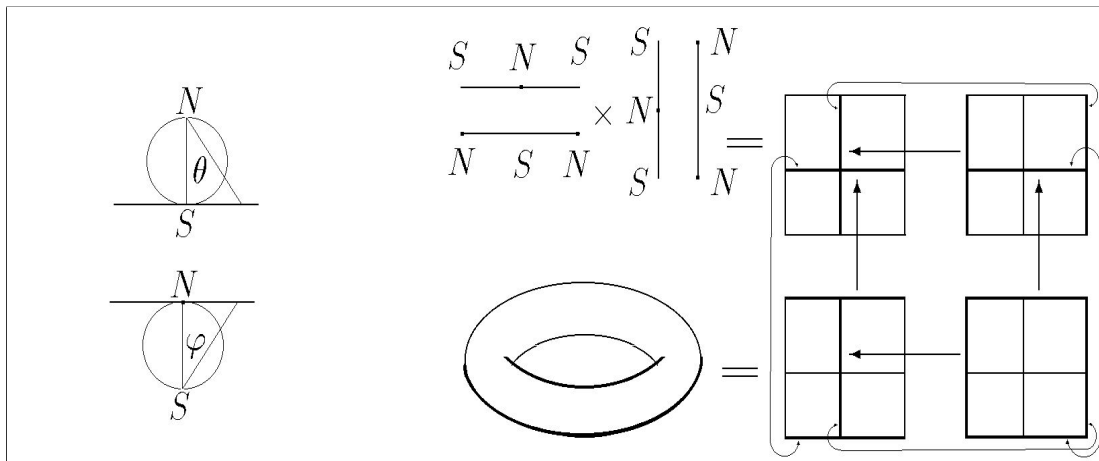
Slika D.1: Atlasi kružnice (levo) i torusa (desno). Svaka od 4 karte torusa nastaje kao proizvod dve karte kružnice. Deblje linije su pri tome nastale od severnog pola na nekoj od karata kružnice, strelice povezuju linije (različitih karata) duž koje treba vršiti "lepljenje" da bi se dobio torus.
